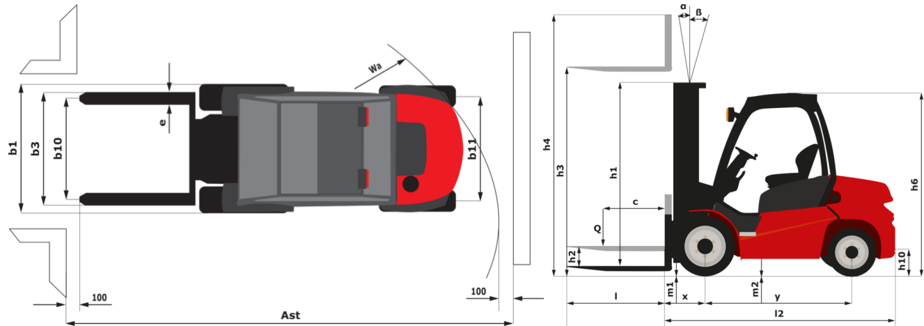
MSI 35 ST5 - Schémas d'encombrement
