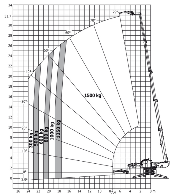
Machine sur stabilisateurs abaissés avec potence 1500 kg
