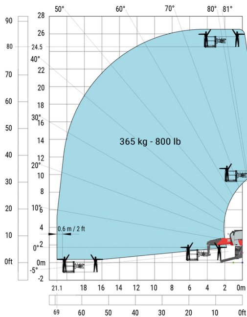
Machine sur stabilisateurs abaissés avec nacelle 365 kg
